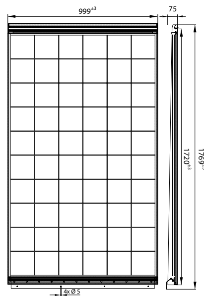
Tutte le misure in mm
